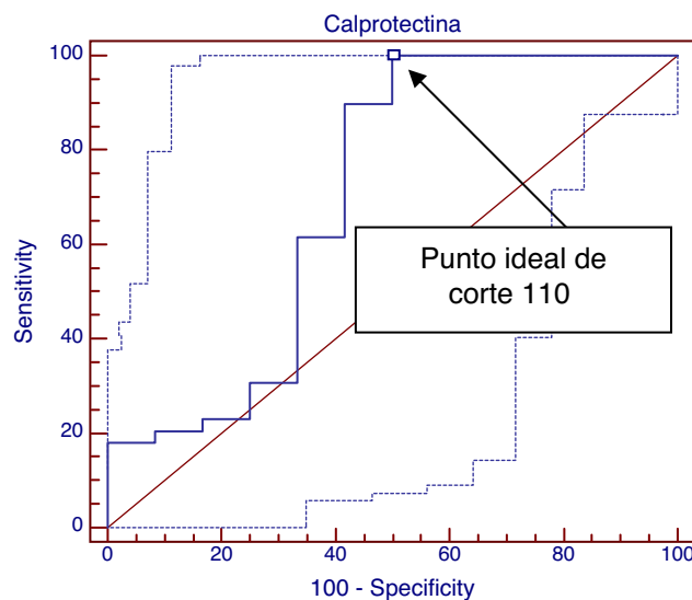
Figura 2 Curva ROC CPF/respuesta clínica positiva al mes. Punto de corte > 110. Sensibilidad 100%, especificidad 50%. Área bajo la curva 0,688, IC 95%: 0,48-0,89.
